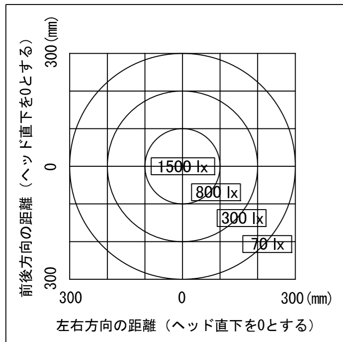
△ 照度分布図
